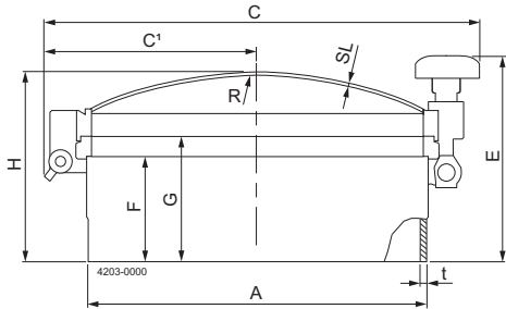
図 2. 寸法
