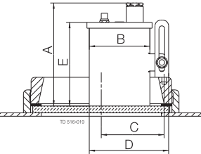
サイト・グラス LKS 105 miniVISION タイプつき 53。
