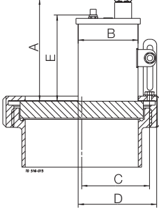
DIN 11851準拠のユニオン・サイト・グラス (miniVision 用) 53。
