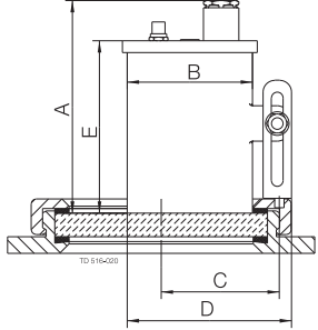
サイト・グラス LKS 78 および 120 miniVISION タイプつき 53。
