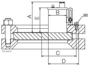
DIN 28120 に準拠したminiVISION 計量タイプのサイト・グラス 53。
