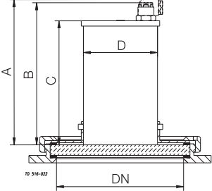
サイト・グラス LKS 78 miniVISION タイプつき 70。
