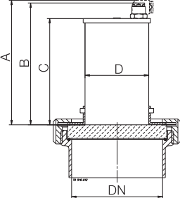
DIN 11851準拠のユニオン・サイト・グラス (miniVision 用) 70。
