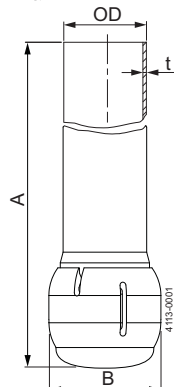
溶接式
