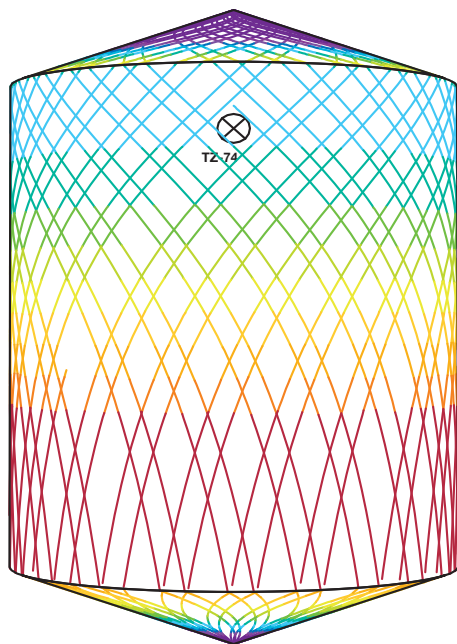
D5m H6m、Toftejorg TZ-74 醸造ケトルバージョン、 4 x ø6 mm、100% Time = 4.4 分、水消費量 = 907 l
